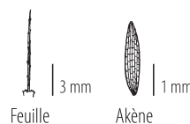
3 – N. gracillima
