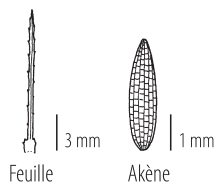
4 – N. indica
